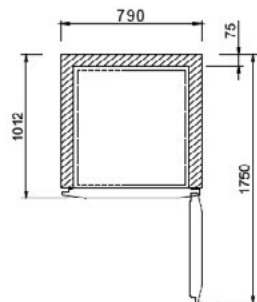
PRALINERIA +4°C +18°C PRELINERY +4°C +18°C
